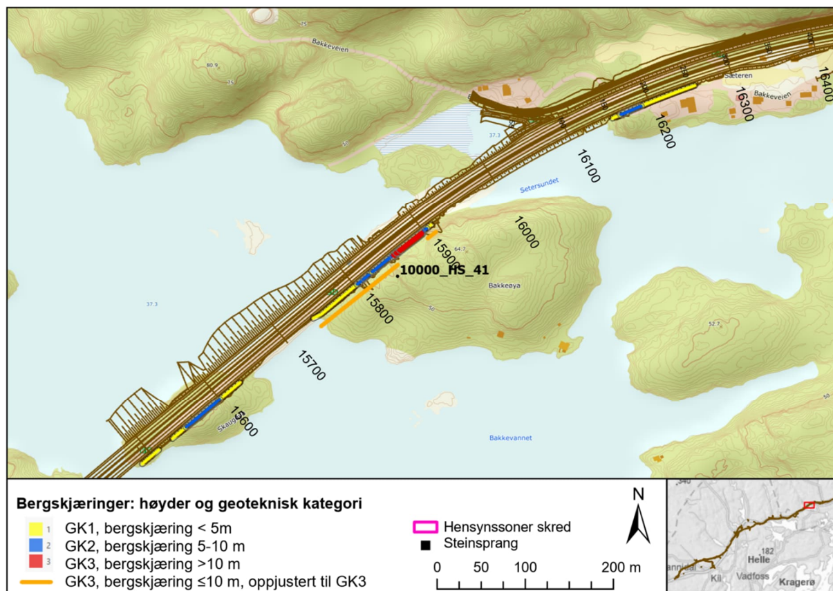
Figur 17-1: Oversikt over bergskjæringer i geoteknisk kategori 1,2 og 3 ved Bakkeøya.
