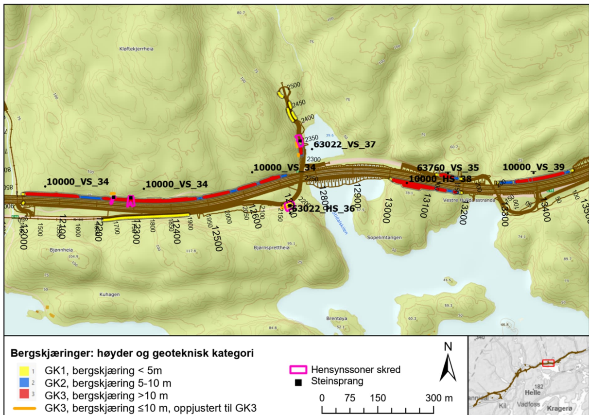
Figur 15-1: Oversikt over bergskjæringer i geoteknisk kategori 1,2 og 3 ved Sopelimtangen.
