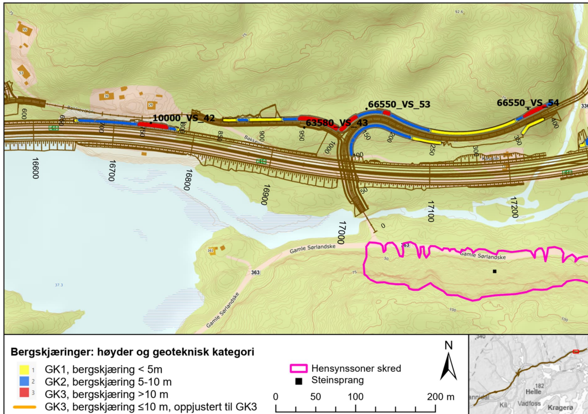
Figur 18-1: Oversikt over bergskjæringer i geoteknisk kategori 1,2 og 3 ved Bakkeveien.
