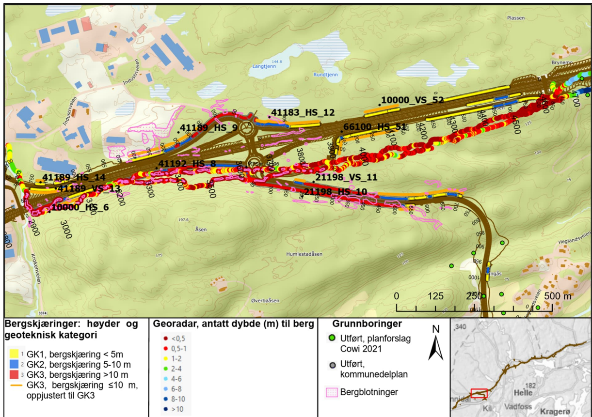
Figur 10-4: Oversikt over utførte grunnundersøkelser i nærheten av bergskjæringer ved Fikkjebakkekrysset.
