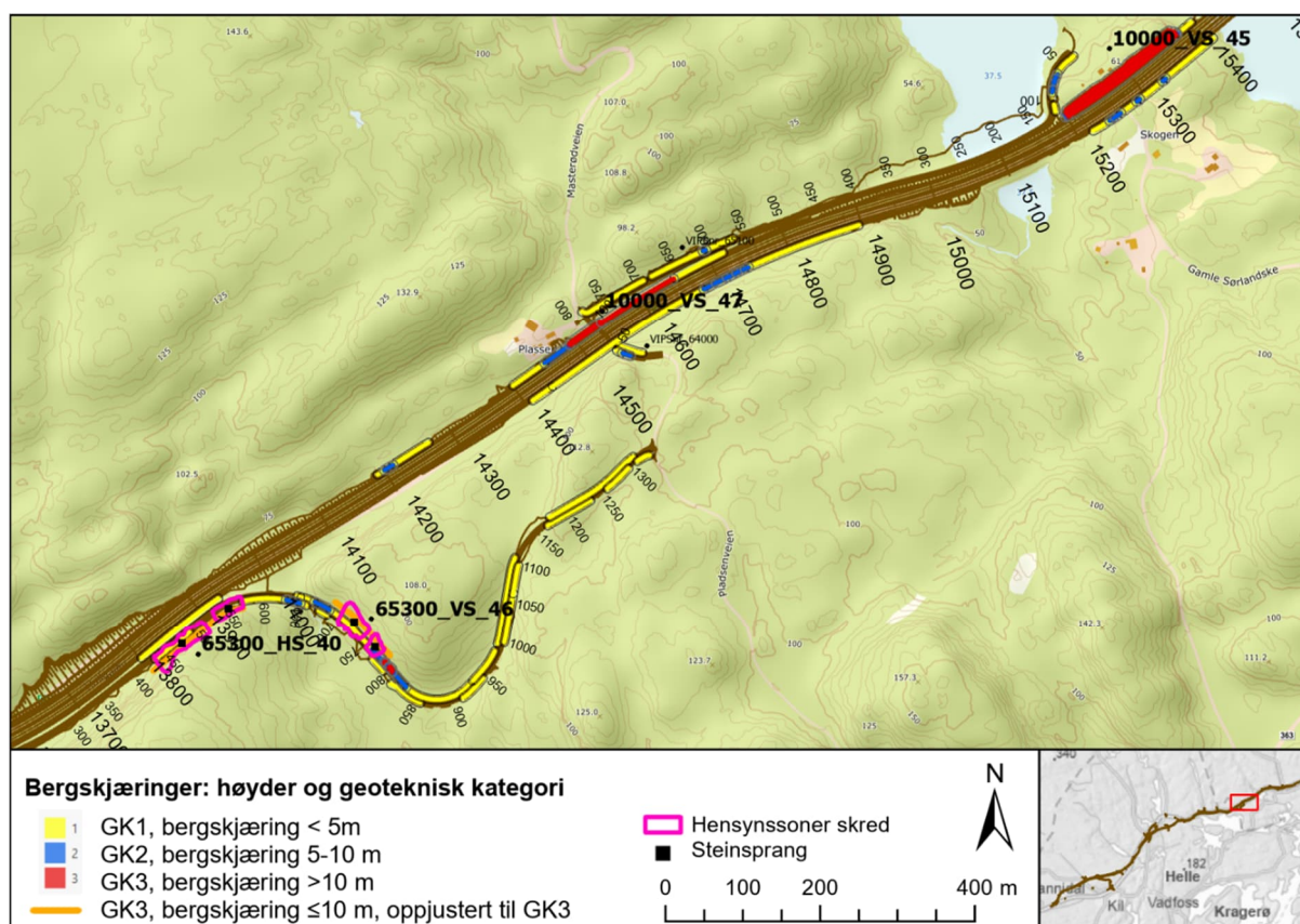
Figur 16-1: Oversikt over bergskjæringer i geoteknisk kategori 1,2 og 3 ved Plassen-Skogen.
