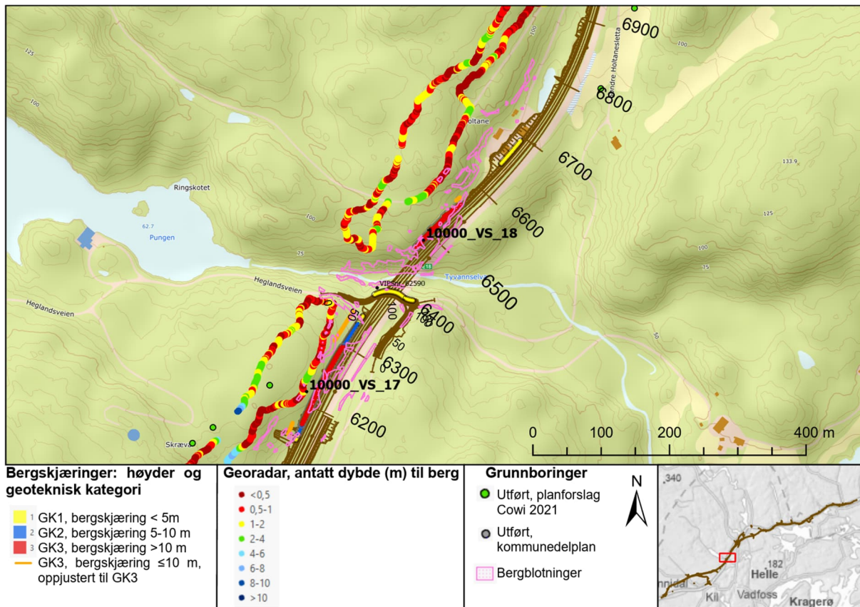
Figur 11-5: Oversikt over utførte grunnundersøkelser ved Hegland-Tyvannselva.
