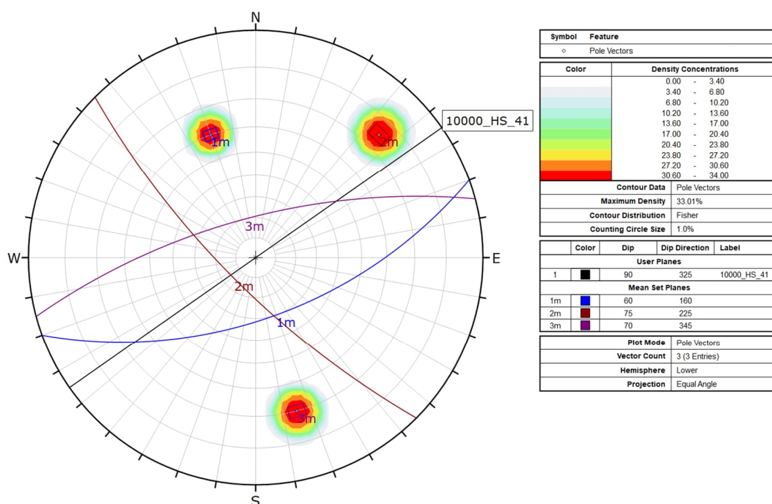
Figur 17-3: Sprekkemålinger (observert fra avstand) registrert i polplott ved Bakkeøya. Linja gjennom sentrum representerer orienteringen av bergskjæringen og er merket med tilhørende skjærings-ID.
