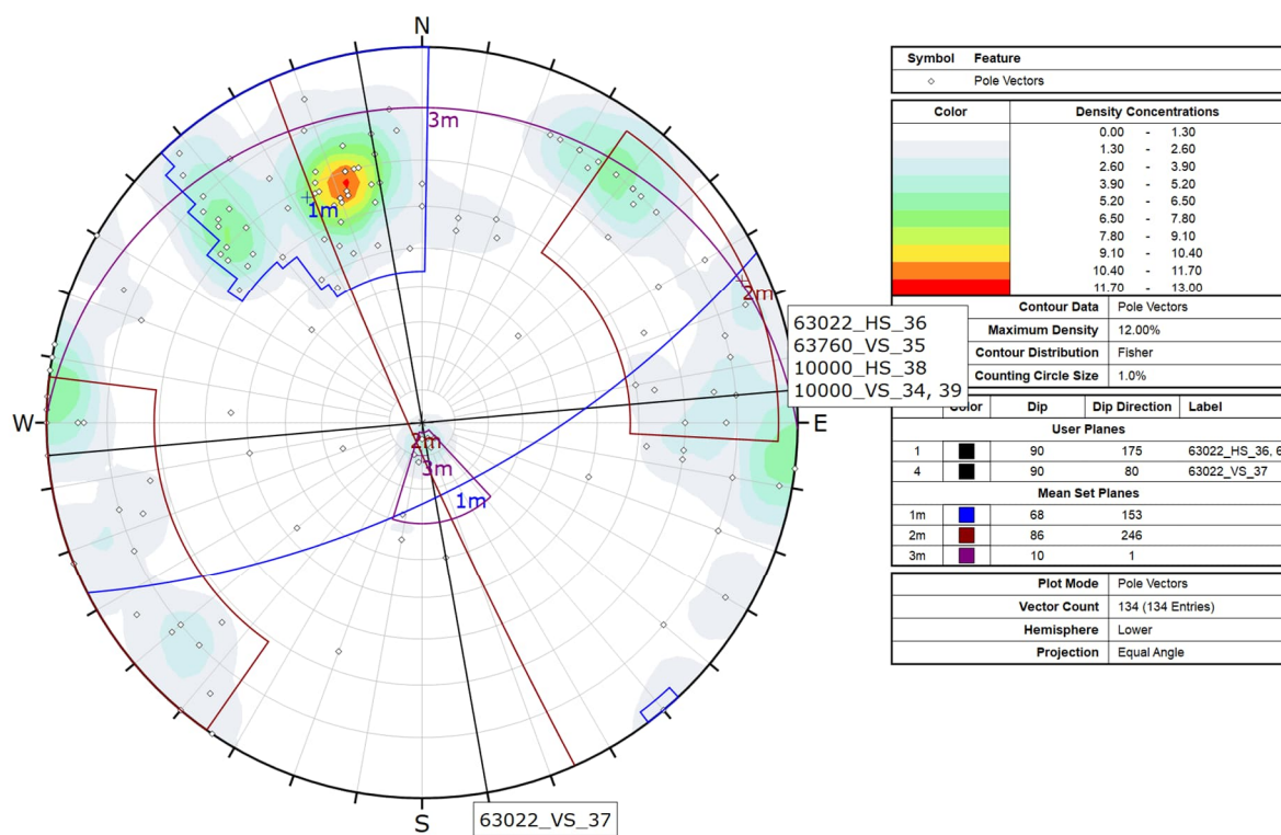
Figur 15-5: Sprekkemålinger som er registrert i polplott ved Sopelimtangen. Linjene gjennom sentrum representerer orienteringen av de ulike bergskjæringene og er merket med tilhørende skjærings-ID.
