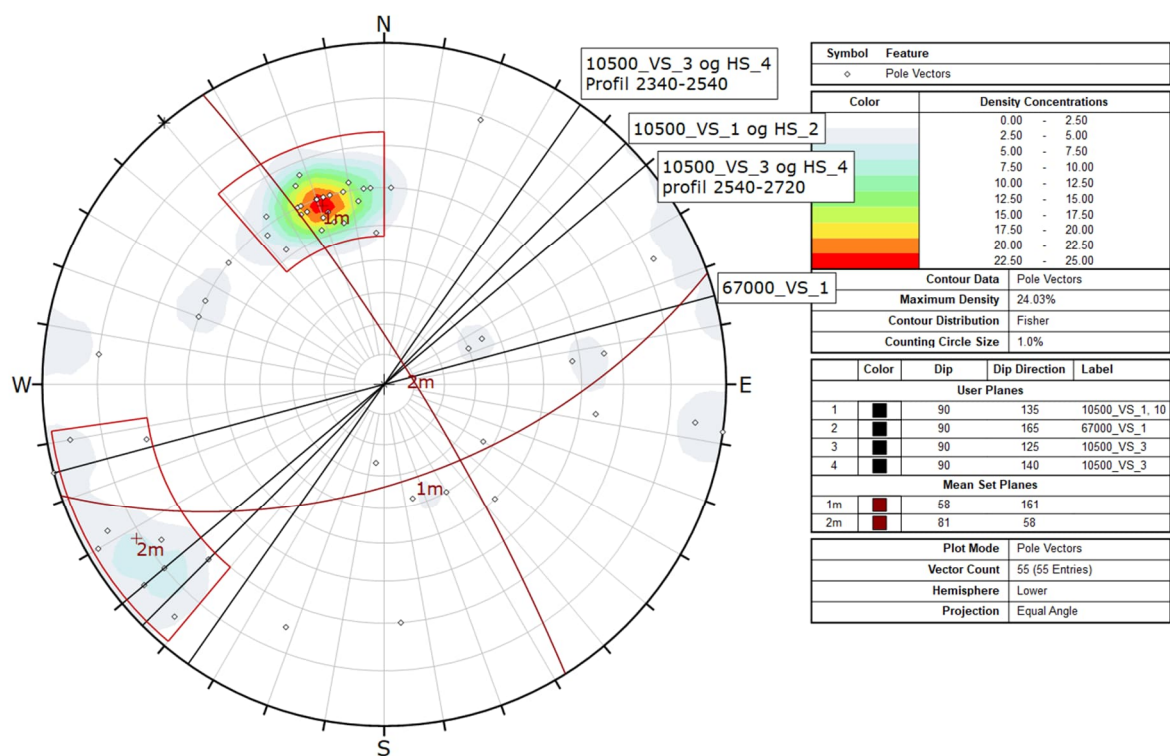
Figur 9-5: Sprekkemålinger som er registrert i polplott ved Dalane-Krokenveien. Linjene gjennom sentrum representerer orienteringen av de ulike bergskjæringene og er merket med tilhørende skjærings-ID.
