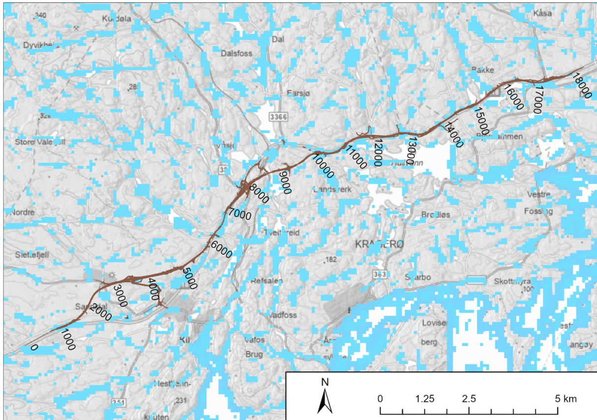
Figur 6-4: Mulige dypforvittringssoner.
