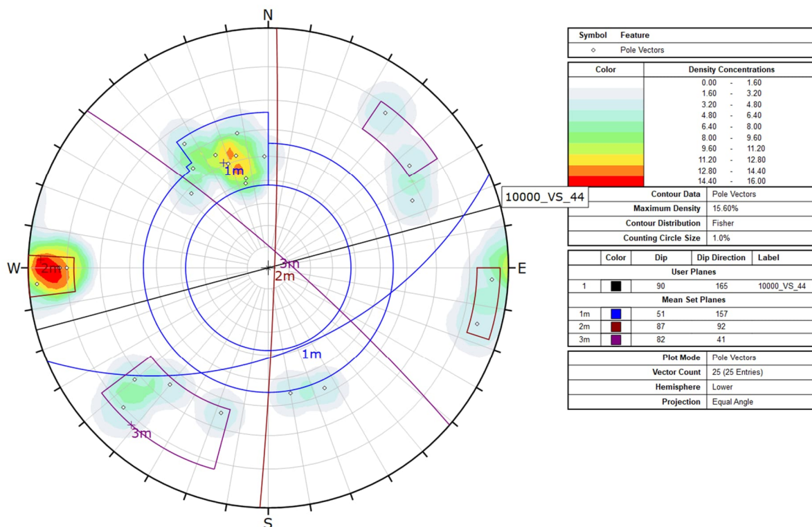
Figur 19-3: Sprekkemålinger som er registrert i polplott ved Dørdal. Linjene gjennom sentrum representerer orienteringen av de ulike bergskjæringene og er merket med tilhørende skjærings-ID.
