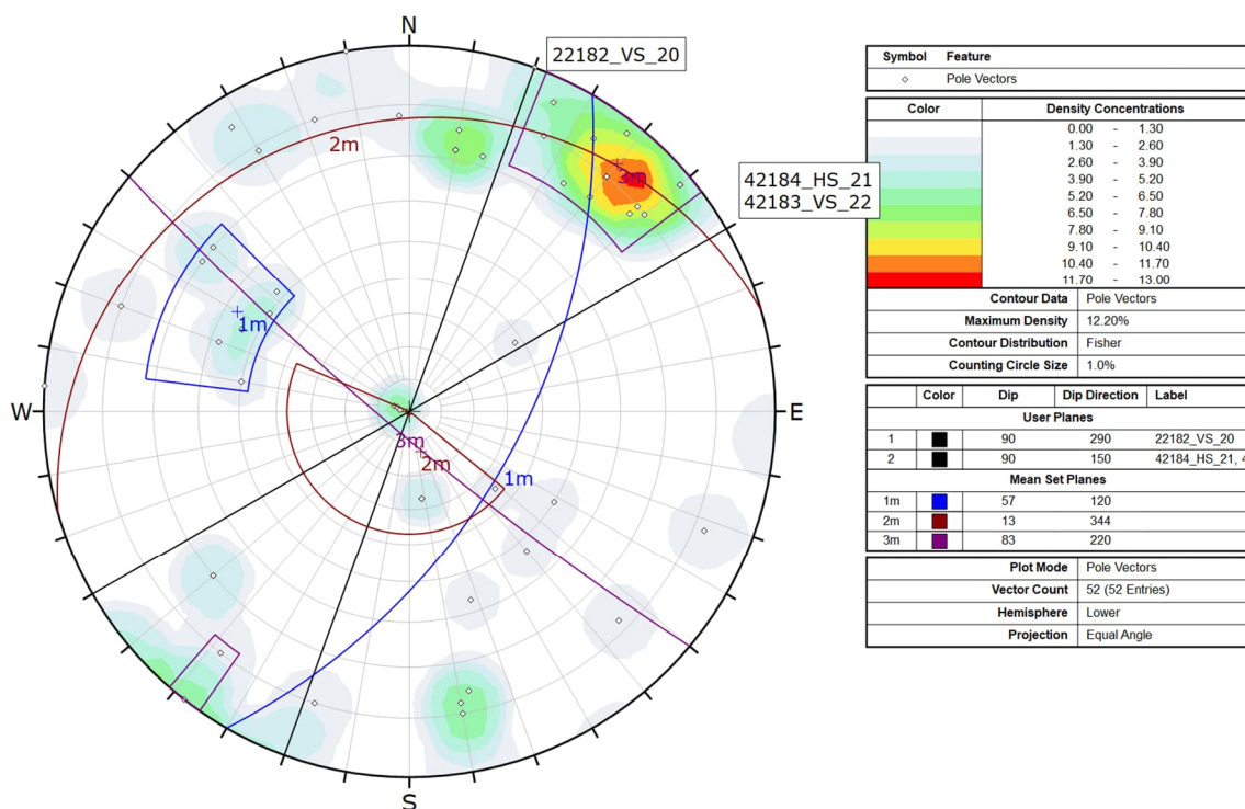
Figur 12-4: Sprekkemålinger som er registrert i polplott ved Gjerdemyrakrysset. Linjene gjennom sentrum representerer orienteringen av de ulike bergskjæringene og er merket med tilhørende skjærings-ID.
