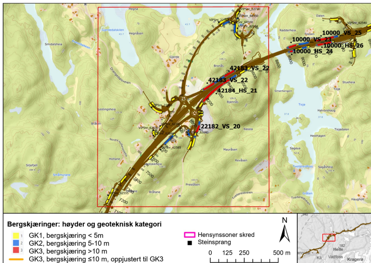
Figur 12-1: Oversikt over bergskjæringer i geoteknisk kategori 1,2 og 3 ved Gjerdemyrakrysset.
