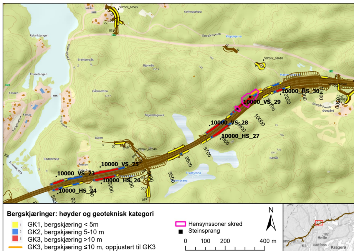
Figur 13-1: Oversikt over bergskjæringer i geoteknisk kategori 1,2 og 3 ved Tisjømyrane.
