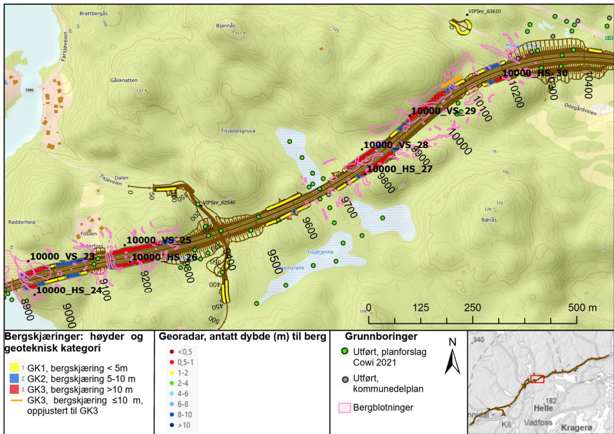
Figur 13-4: Oversikt over utførte grunnundersøkelser ved Tisjømyrane.
