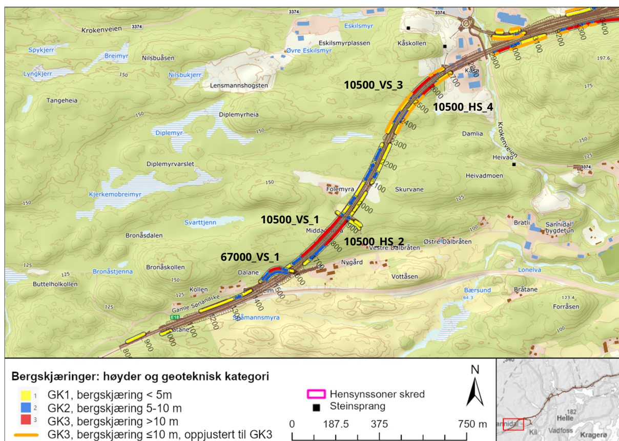
Figur 9-1: Oversikt over bergskjæringer i geoteknisk kategori 1,2 og 3 ved Dalane-Krokenveien.
