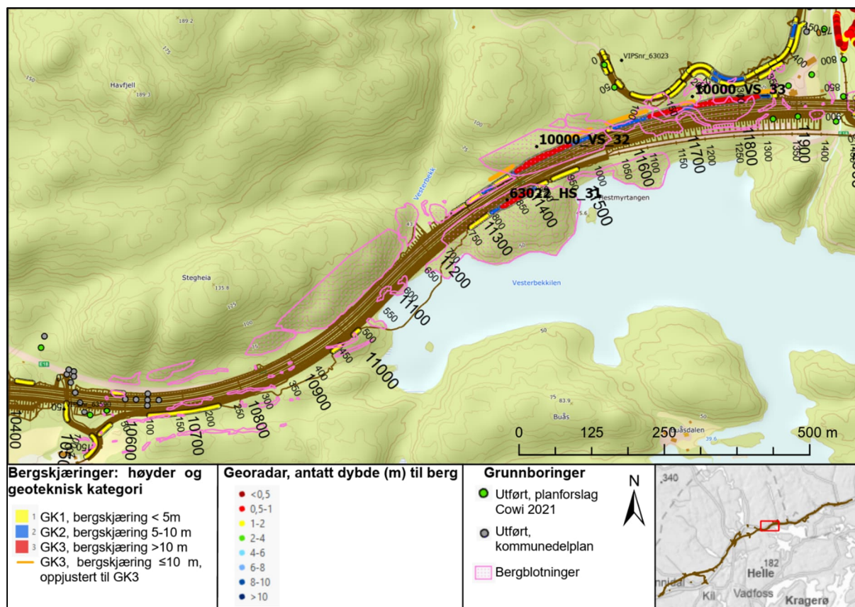
Figur 14-3: Oversikt over utførte grunnundersøkelser ved Vesterbekkilen.
