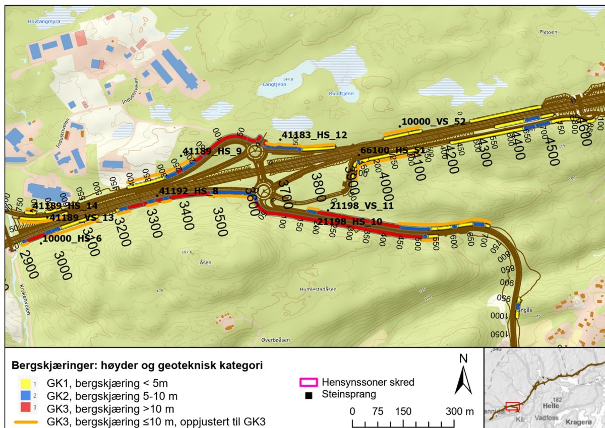
Figur 10-1: Oversikt over bergskjæringer i geoteknisk kategori 1,2 og 3 ved Fikkjebakkekrysset.
