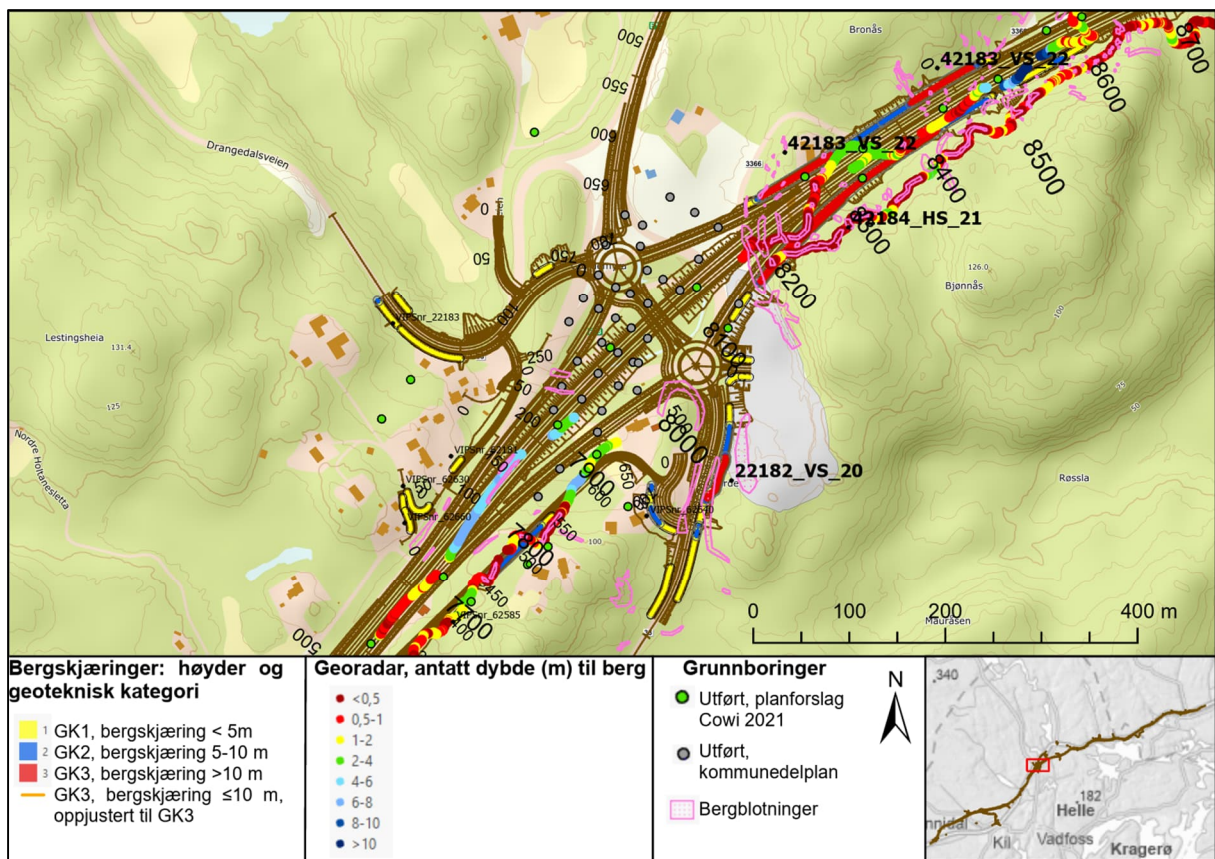
Figur 12-3: Oversikt over utførte grunnundersøkelser i Gjerdemyrakrysset.
