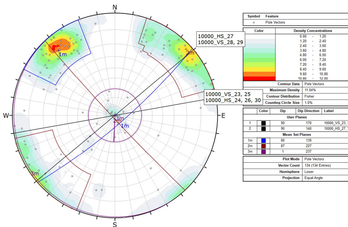
Figur 13-5: Sprekkemålinger som er registrert i polplott ved Tisjømyrane. Linjene gjennom sentrum representerer orienteringen av de ulike bergskjæringene og er merket med tilhørende skjæring-ID.
