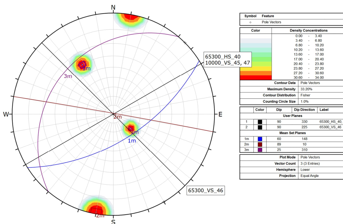
Figur 16-7: Sprekkeretninger observert fra avstand, vist som polplott ved Plassen-Skogen. Linjene gjennom sentrum representerer orienteringen av de ulike bergskjæringene og er merket med tilhørende skjærings-ID.
