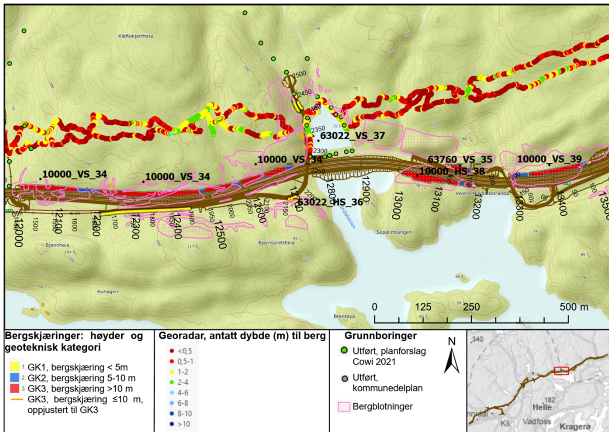
Figur 15-4: Oversikt over utførte grunnundersøkelser ved Sopelimtangen.
