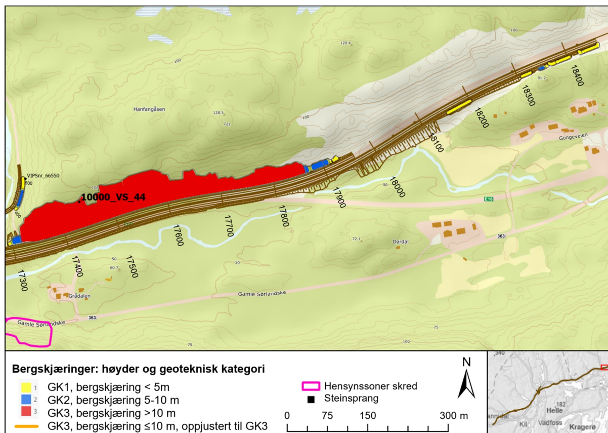
Figur 19-1: Oversikt over bergskjæringer i geoteknisk kategori 1,2 og 3 ved Dørdal.
