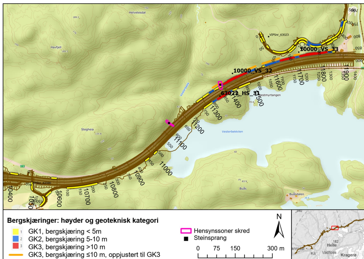
Figur 14-1: Oversikt over bergskjæringer i geoteknisk kategori 1,2 og 3 ved Vesterbekkilen.
