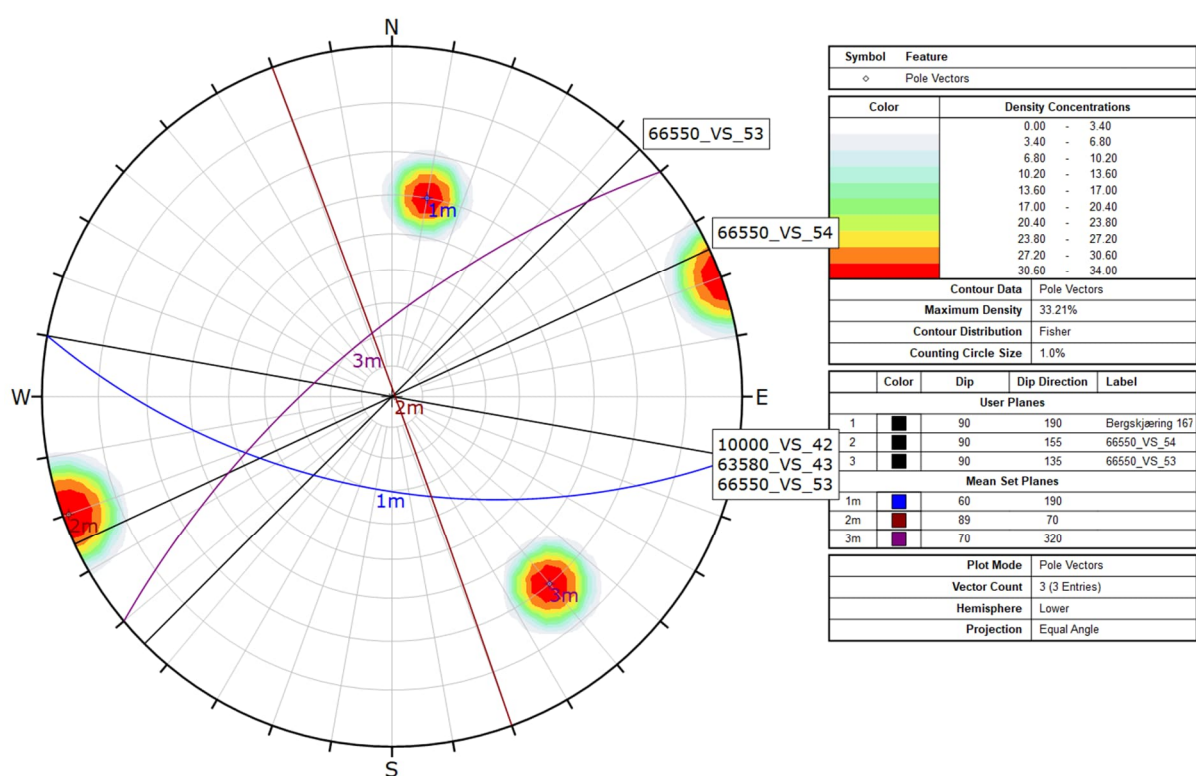
Figur 18-3: Sprekkemålinger (observert fra avstand) i polplott ved Bakkeveien. Linjene gjennom sentrum representerer orienteringen av de ulike bergskjæringene og er merket med tilhørende skjærings-ID.
