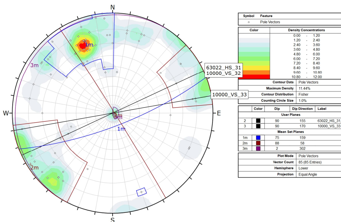
Figur 14-4: Sprekkemålinger som er registrert i polplott ved Vesterbekkilen. Linjene gjennom sentrum representerer orienteringen av de ulike bergskjæringene og er merket med tilhørende skjærings-ID.
