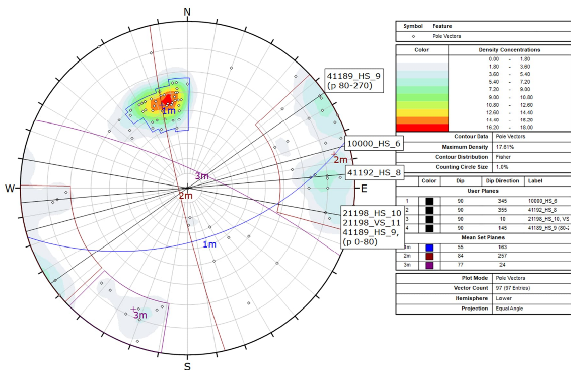
Figur 10-5: Sprekkemålinger som er registrert i polplott ved Fikkjebakkekrysset. Linjene gjennom sentrum representerer orienteringen av de ulike bergskjæringene og er merket med tilhørende skjærings-ID.
