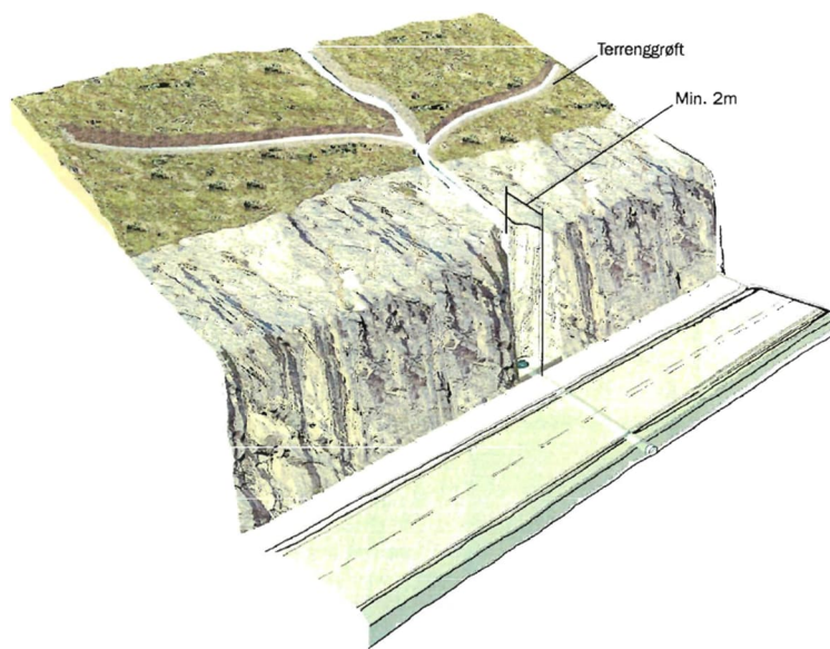
Figur 5-2: Prinsippskisse terrenggrøfter og nisje i skjæring (illustrasjon hentet fra [30]).
