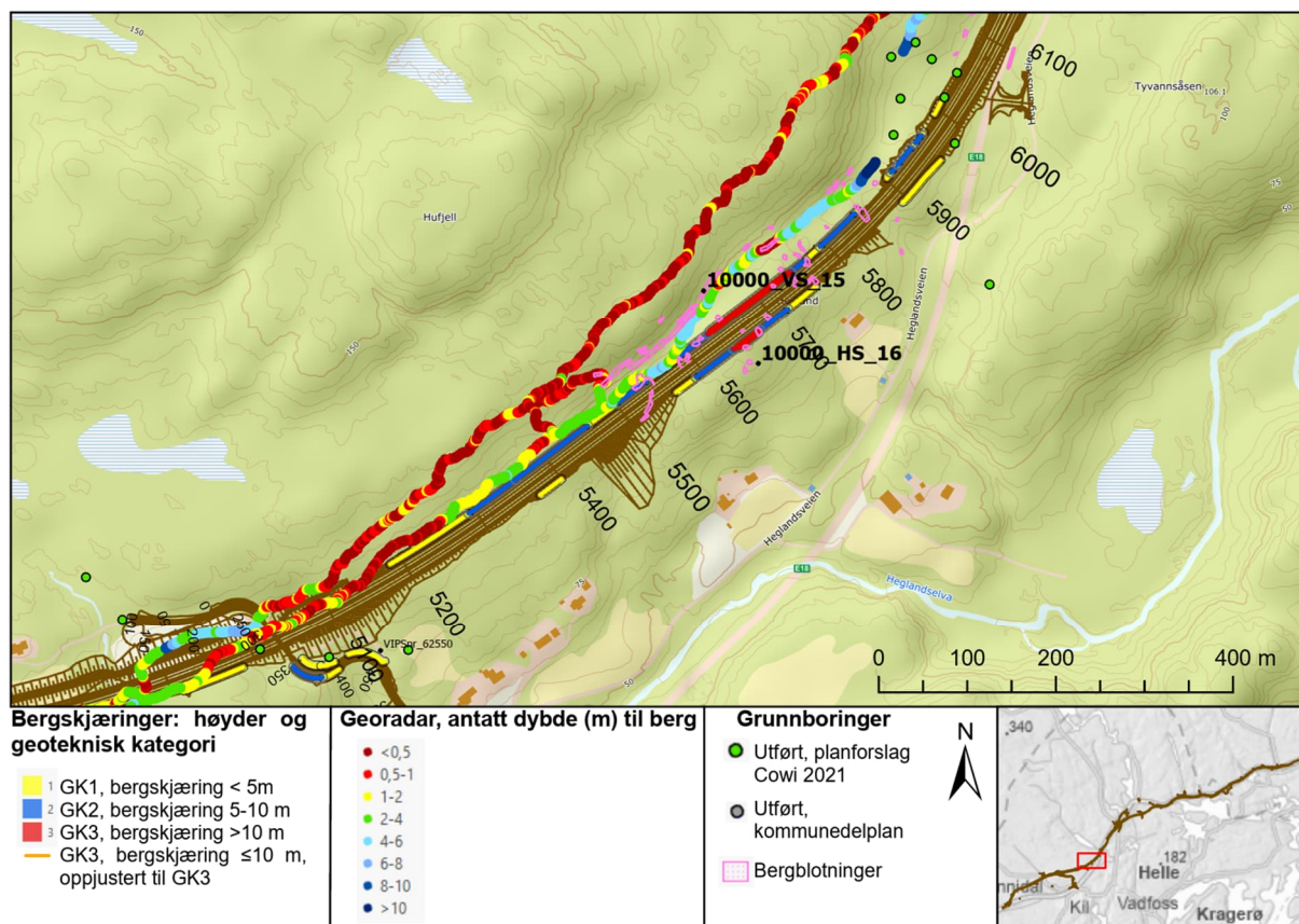
Figur 11-4: Oversikt over utførte grunnundersøkelser ved Hegland-Tyvannselva.
