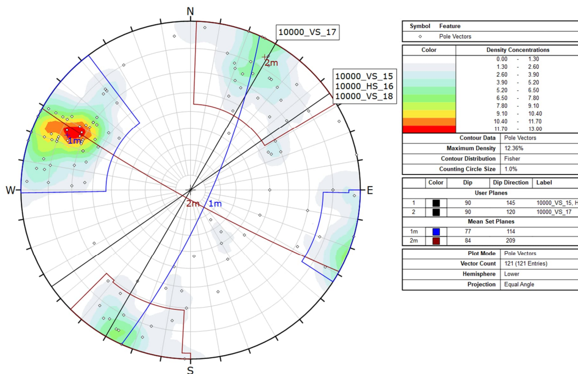
Figur 11-6: Polplott: Sprekkemålinger som er registrert i polplott ved Hegland-Tyvannselva. Linjene gjennom sentrum representerer orienteringen av de ulike bergskjæringene og er merket med tilhørende skjærings-ID.
