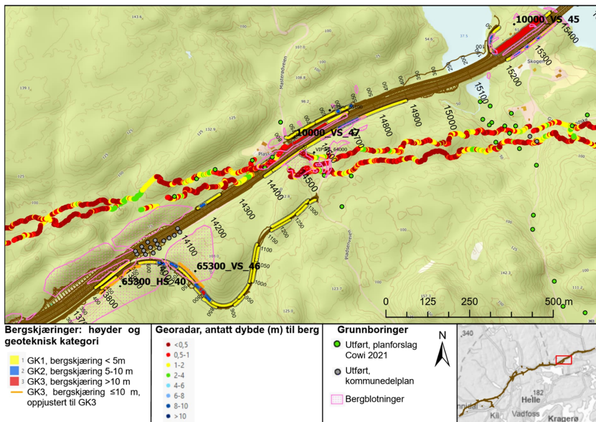
Figur 16-6: Oversikt over utførte grunnundersøkelser ved Plassen-Skogen.
