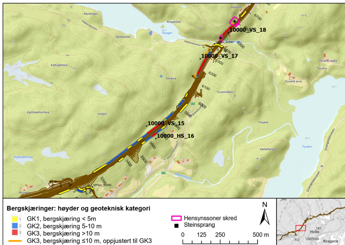
Figur 11-1: Oversikt over bergskjæringer i geoteknisk kategori 1,2 og 3 ved Hegland-Tyvannselva.
